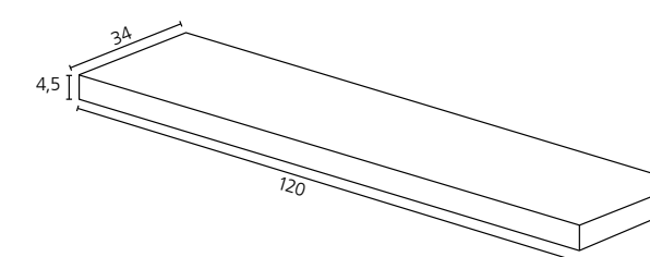
ANGOLARE DX GRADINO PLUS** 34x120x4,5 cm RECT - 13 3 / 8 "x48x1 3 / 4 " LUX* ± 10 mm
